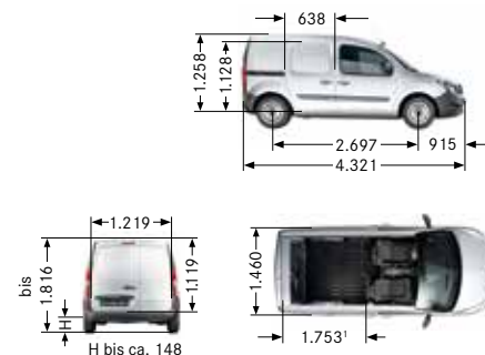
Kastenwagen lang mit 2.697 mm Radstand
