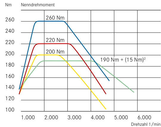
Drehmomentverläufe:
