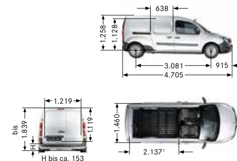
Kastenwagen extralang mit 3.081 mm Radstand
