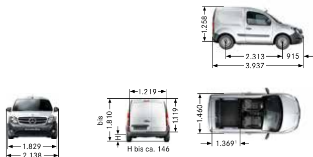
Kastenwagen kompakt mit 2.313 mm Radstand
